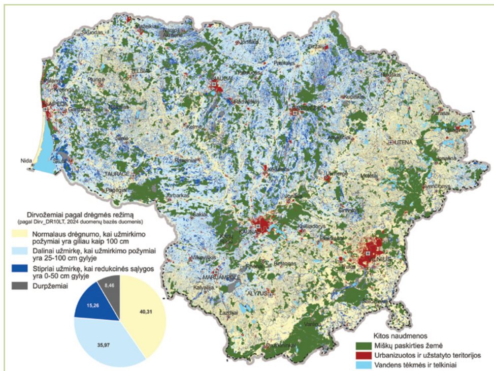
(4.11. pav. Užmirkusių dirvožemių paplitimas Lietuvoje (J. Volungevičius, 2026).)
