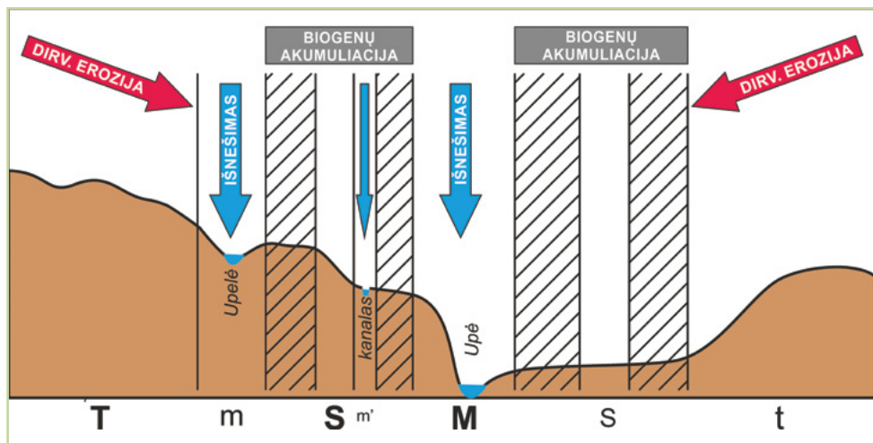
(5.1. pav. Intensyvaus ūkininkavimo agroekosistema su gamtinio karkaso elementais, jų neįveikiant, schema. (Gamtinio karkaso ruožai agroekosistemoje pažymėti: T, t – regioninės ir vietinės svarbos geoeekologinės takoskyros, M, m, m' – regioninės, rajoninės ir vietinės svarbos migracijos koridoriai, S, s – regioninės ir vietinės svarbos vidinio stabilizavimo arealai. I, II, III – tausojančio ūkininkavimo, kraštotvarkos ir agromiškininkystės priemonių sąlyginės grupės.)
