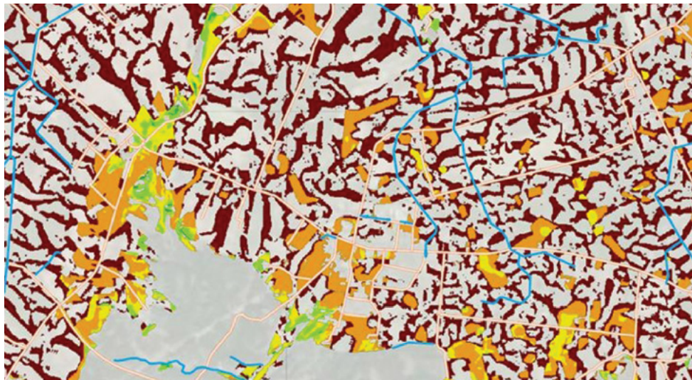
(5.4.pav. Medynų įveisimui tinkamų plotų atsižvelgiant į sausinamosios melioracijos sistemų išsidėstymą, identifikavimas)
