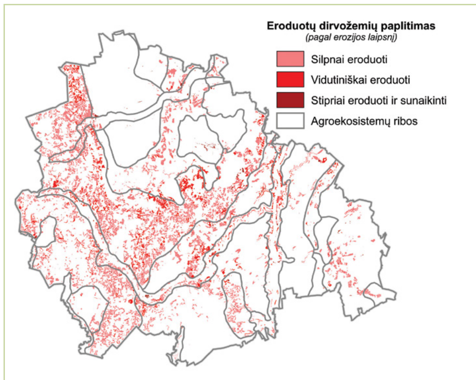
(5.7. pav. Eroduotų dirvožemių erdvinė sklaida Kelmės r. sav. teritorijos žemės ūkio naudmenose)
