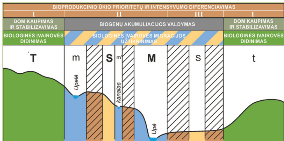
(5.2. pav. Tausojančio (buvusio intensyvaus) ūkininkavimo agroekosistema su gamtinio karkaso elementais, juos įveiklinus, schema. Gamtinio karkaso ruožai agroekosistemoje pažymėti: T, t – regioninės ir vietinės svarbos geoeekologinės takoskyros, M, m, m' – regioninės, rajoninės ir vietinės svarbos migracijos koridoriai, S, s – regioninės ir vietinės svarbos vidinio stabilizavimo arealai. I, II, III – tausojančio ūkininkavimo, kraštotvarkos ir agromiškininkystės priemonių sąlyginės grupės.)
