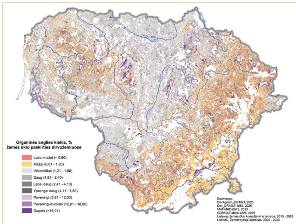
(4.13. pav. Organinės anglies kiekis žemės ūkio paskirties dirvožemiuose (J. Volungevičius, 2025))
